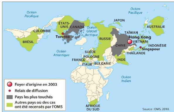
Doc. 1 La diffusion du SRAS (syndrome respiratoire aigu sévère)
